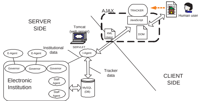
Fig. 3. Human - eI interaction
